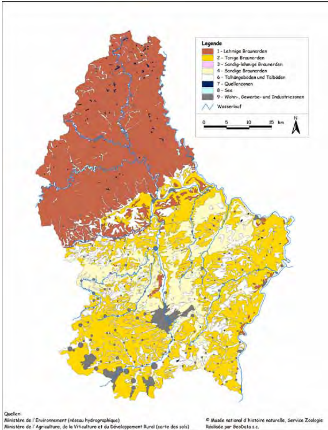
Abb. 8: Bodentypen des Großherzogtums Luxemburgs.
