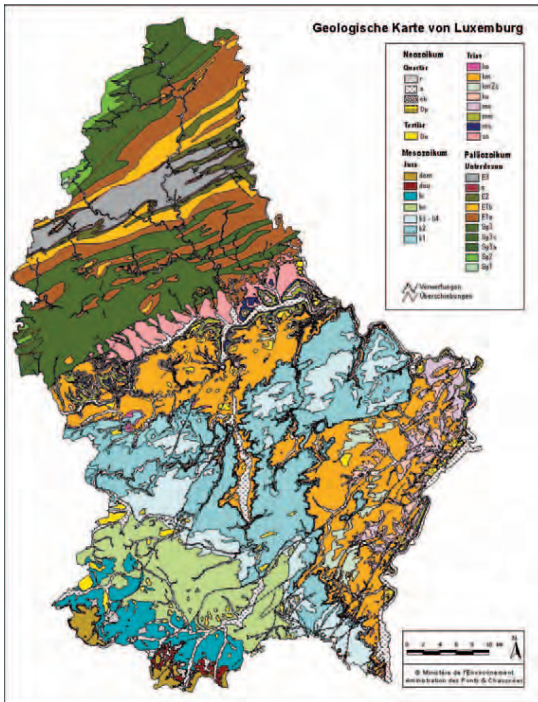
Abb. 7: Geologie des Großherzogtums Luxemburgs.
