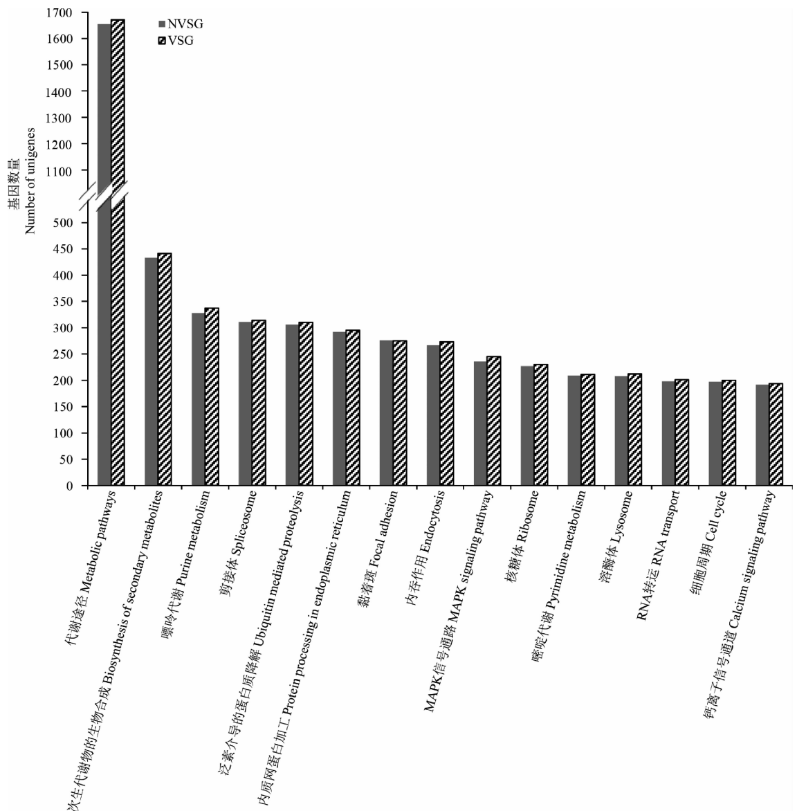
图 4 白背飞虱唾液腺 unigenes 的 KEGG 通路分布
