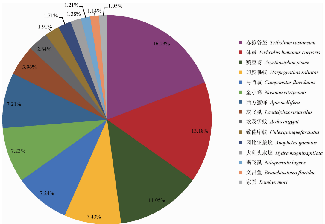
图2 白背飞虱唾液腺 unigenes 同源序列在 NR 数据库注释的物种分布图
